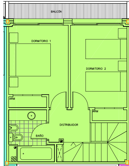
PLANTA PRIMERA
